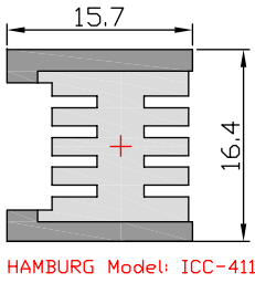
HAMBURG Model: ICC-411
