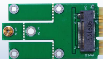
M2MU2 (M.2 (NGFF) - USB タイプ mPCIe アダプタ) x1
